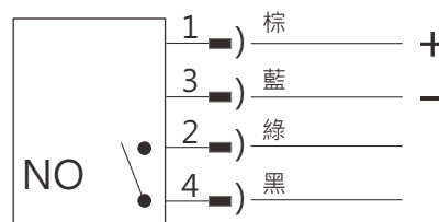
圖 10 繼電器輸出型(NO)
