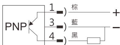
圖 8 PNP輸出型
