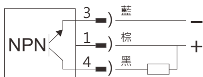
圖 7 NPN輸出型
