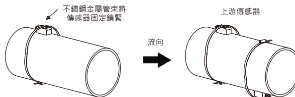
Z型安裝(圖3)
